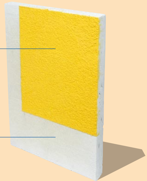
Leichtgrundputz 2 cm
